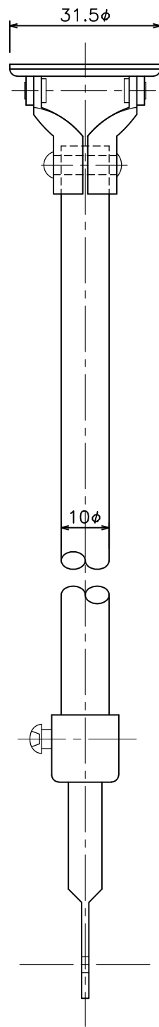
R天井吊棒(伸縮角度自由)(5T9※)
