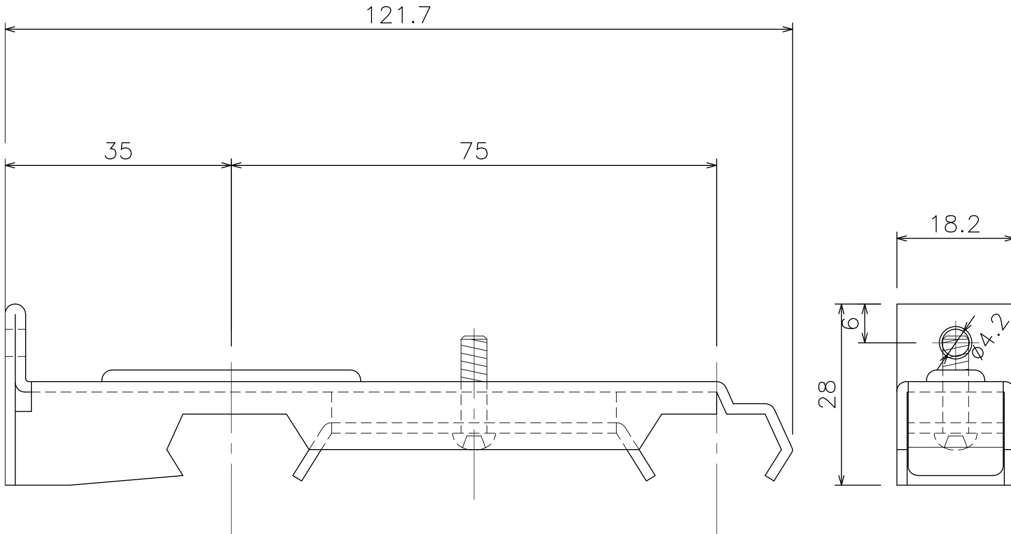
C型 ロングWブラケット (1T46) (住宅公団AI-911C1型用)
