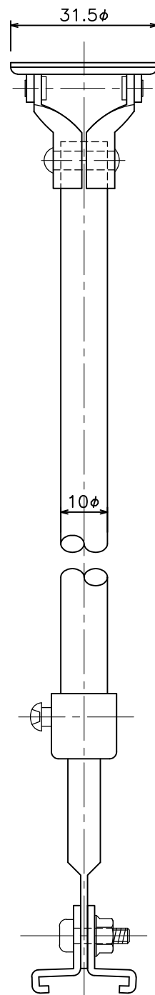
ダンディー 天井吊棒(伸縮角度自由)(2T9※)
