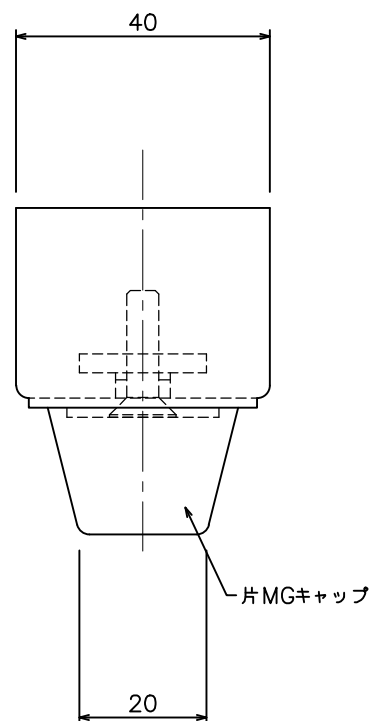
D40片マグネットランナー(片開)ステージランナー (15Y32)
