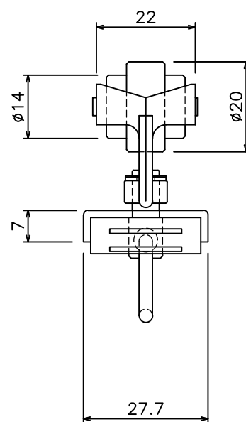
D40片マグネットランナー(片開)ステージランナー (15Y32)
