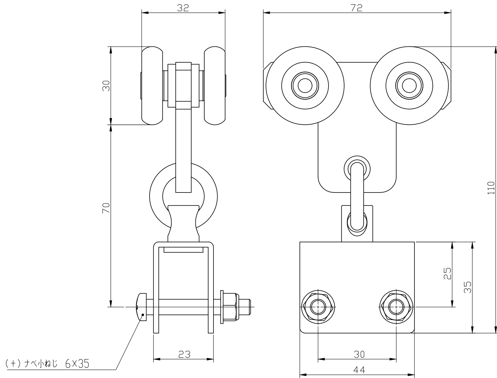
SG間仕切ランナーN (27T28N)
