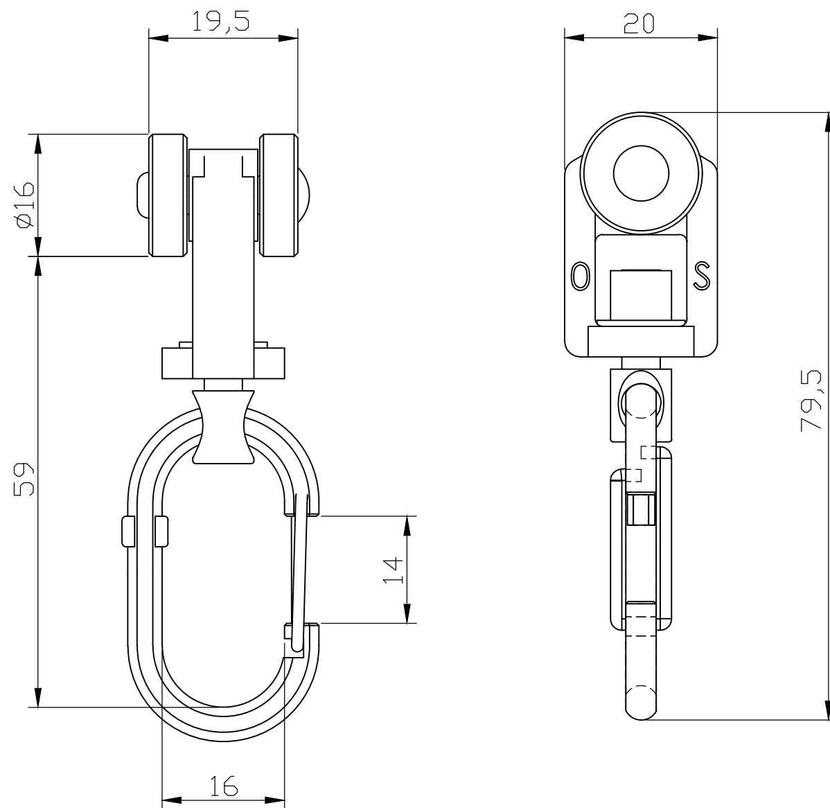
D40ベアリング入ワンタッチランナー (15T27)
