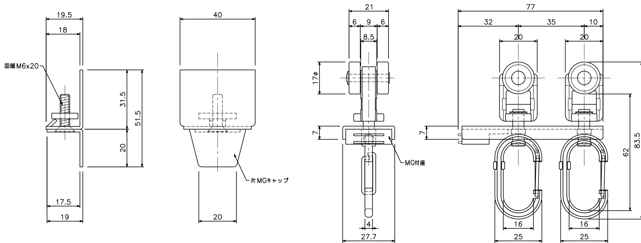
D40片マグネットランナー (片開)ワンタッチランナーA (15Y33)
