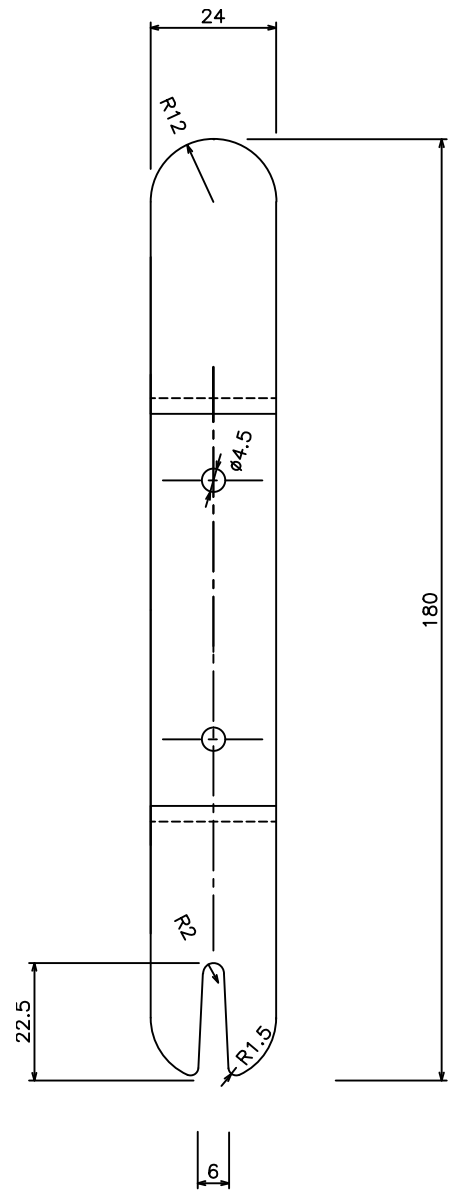
紐掛け (76T92)
