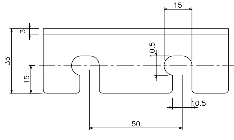
ステンADWブラケット ( 76T46 )
