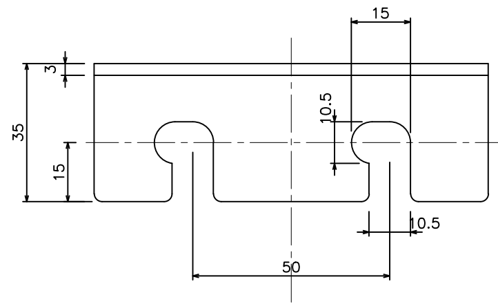
ADWブラケット ( 76T45 )
