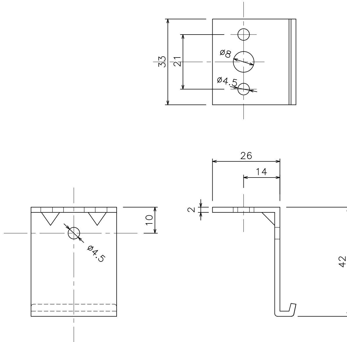
ステンADブラケット (76T44)
