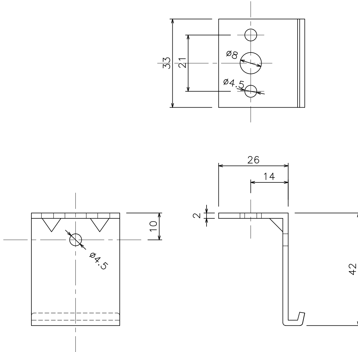
ADブラケット (76T43)
