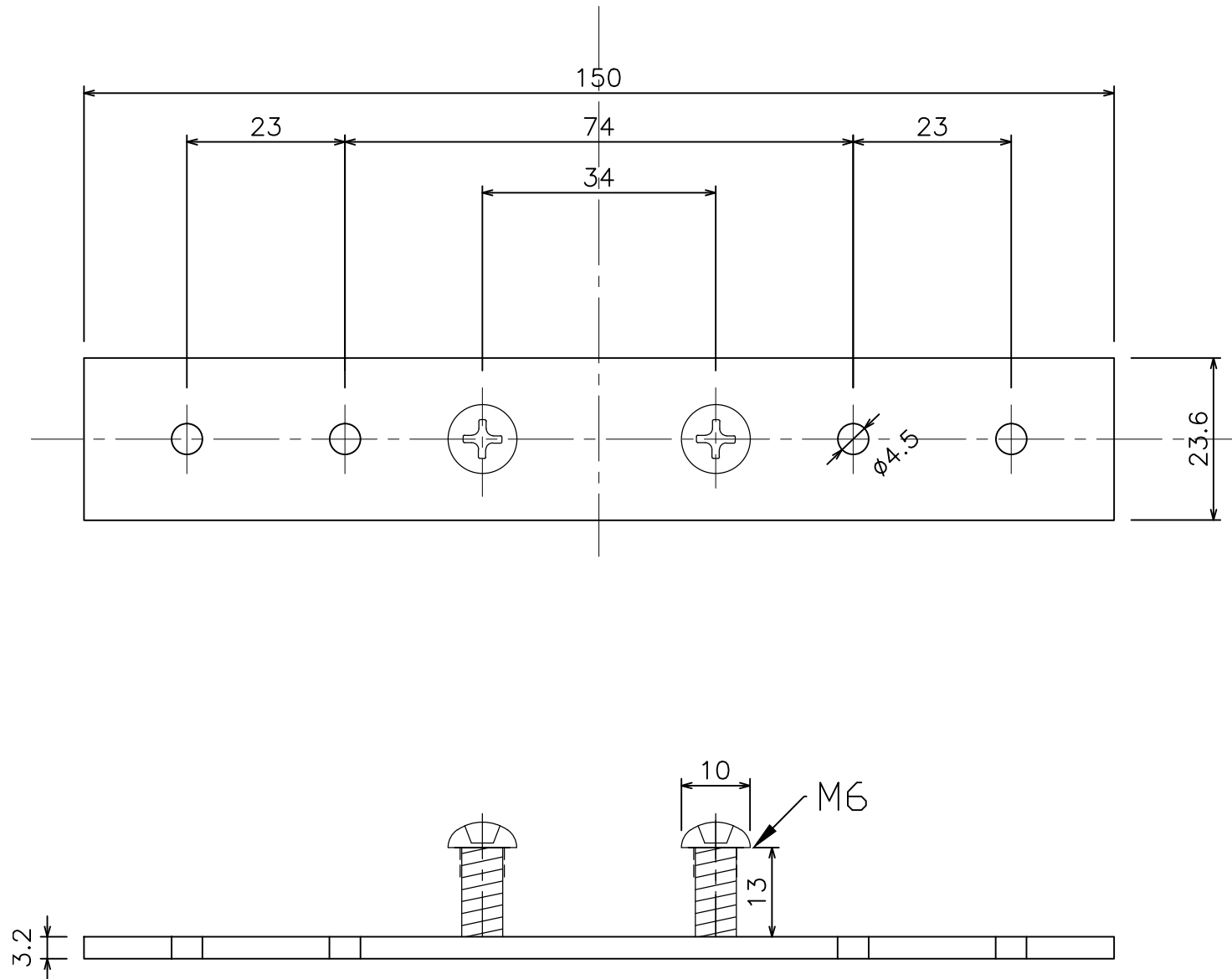
ステン横棧Wシート留め金具 (76T66)
