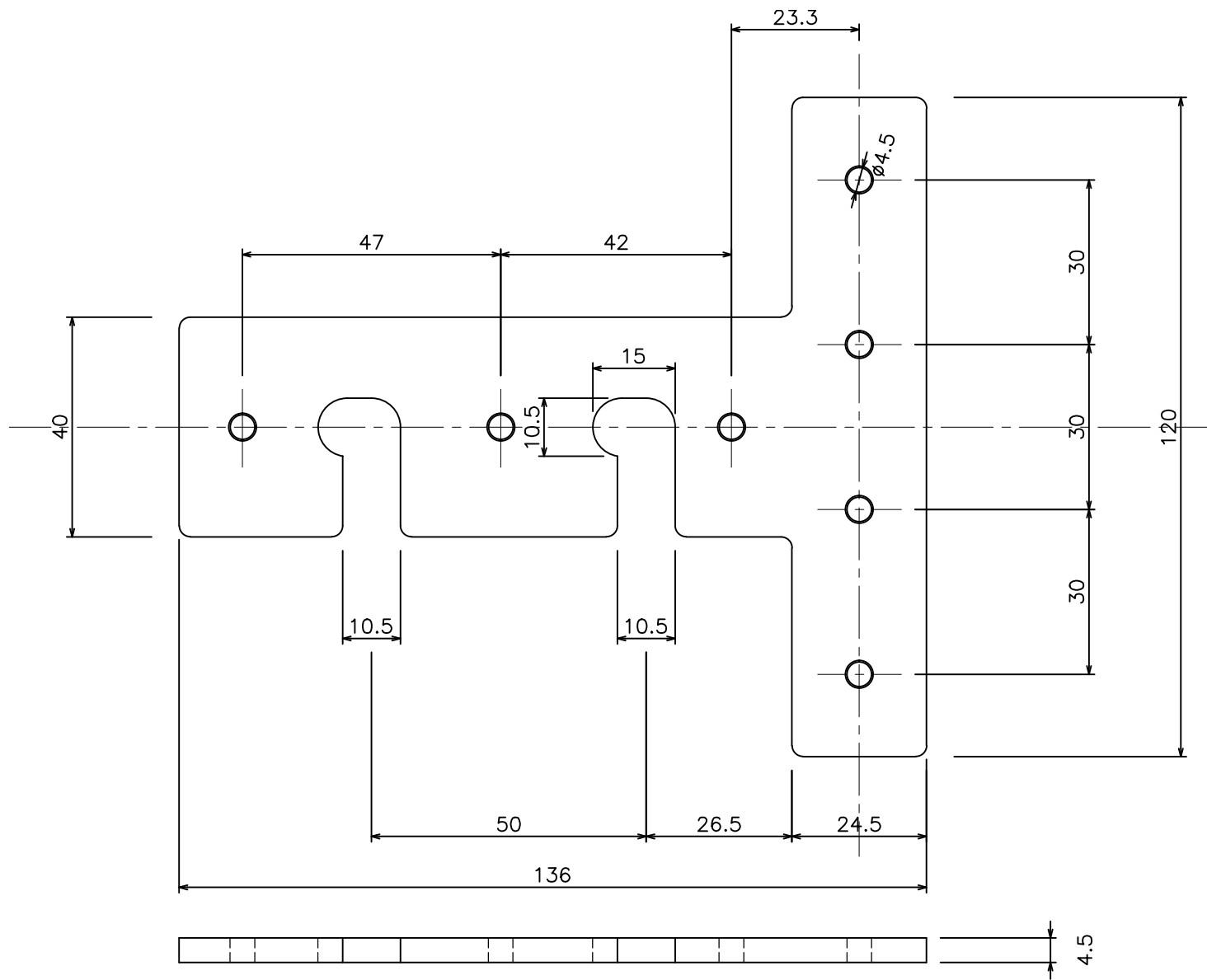
ステン横棧T型取付金具 (76T58)
