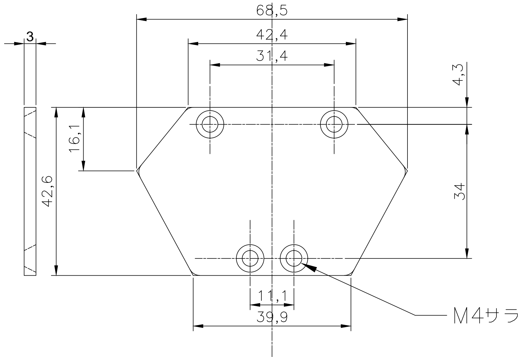
ADWキャッププレート (76T37)
