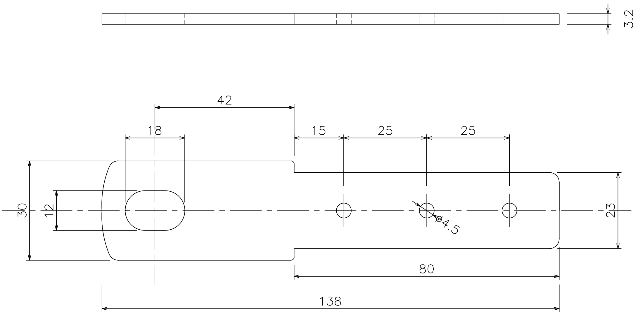
可動バー取付金具 (76T69)
