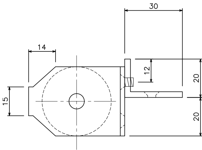
ステン水平用S滑車 (76T76)
