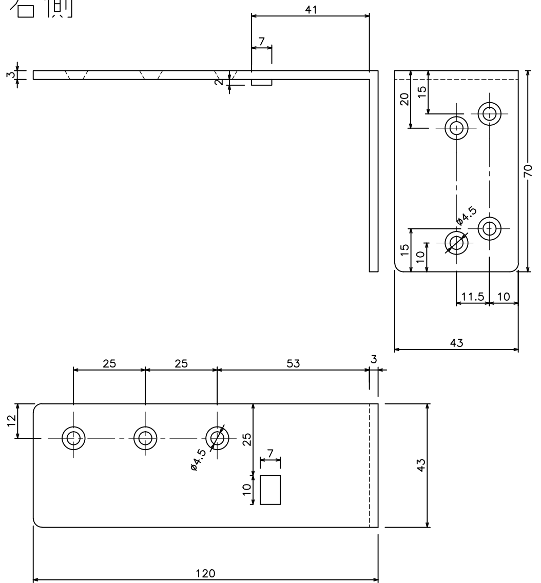
ステン横棧L型取付金具 (76T56)
