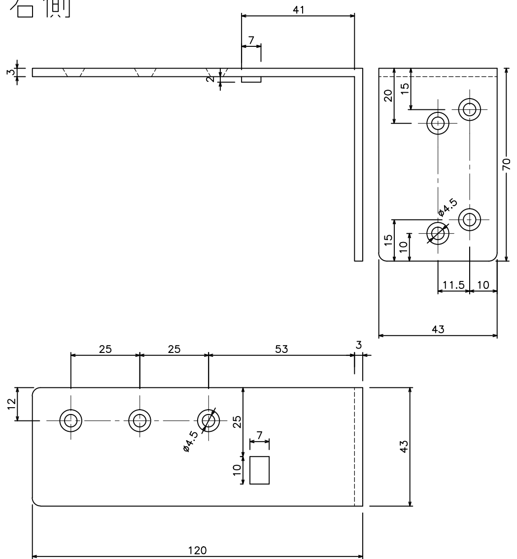
横棧L型取付金具 (76T55)
