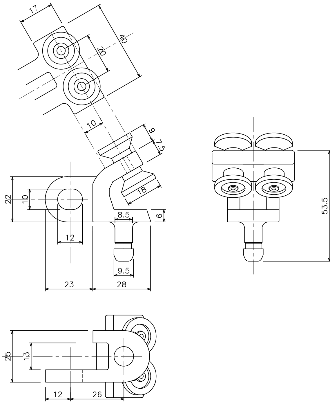
ADランナー (76T11)
