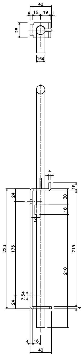
間仕切 落とし16φボルト式 (90T76)
