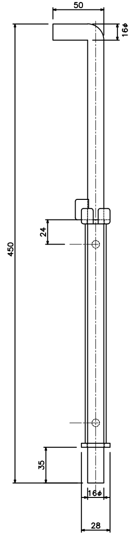
間仕切 落とし16φボルト式 (90T76)
