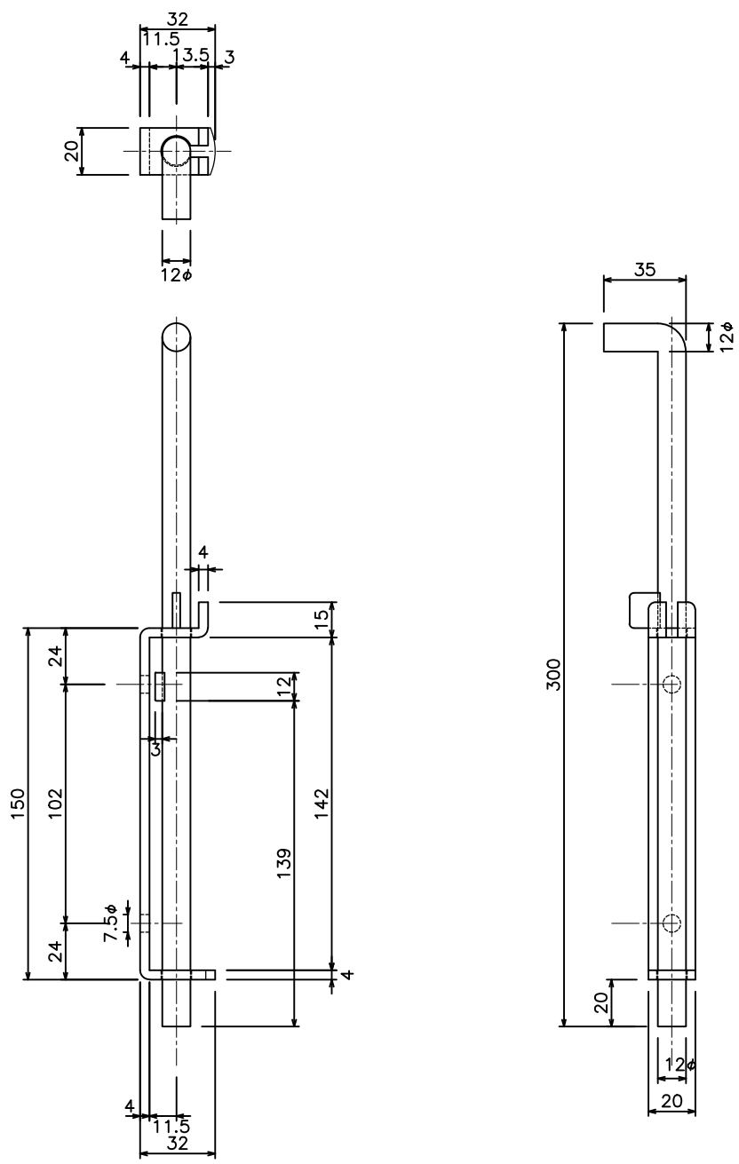
間仕切 落とし12φボルト式 (90T73)
