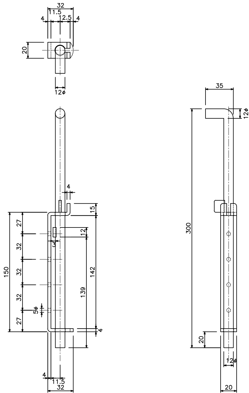
問仕切 落とし12φビス式 (90T71)
