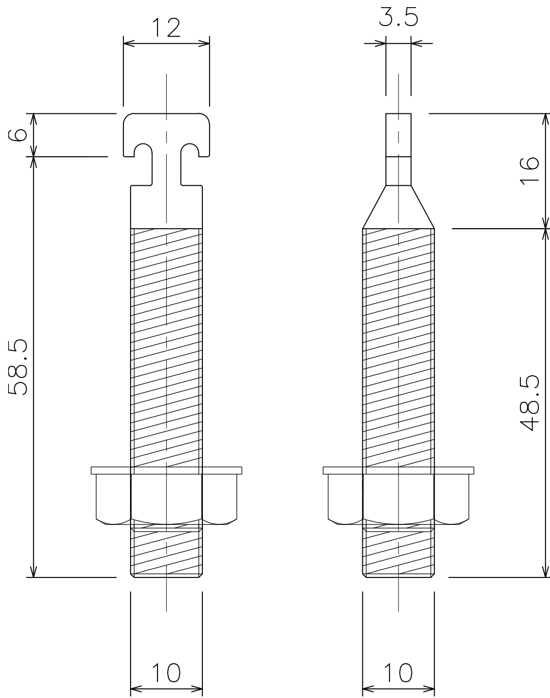
テンションボルト B (81T92)
