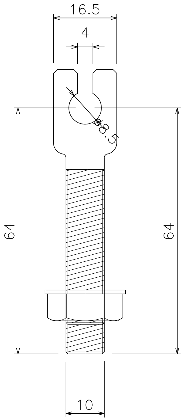
テンションボルト A (81T91)
