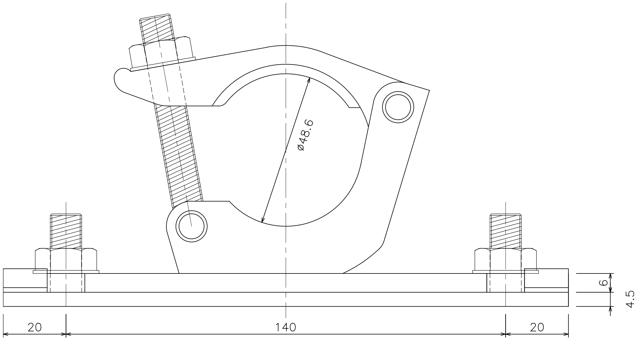
開閉シートクランプ付ブラケット (26T41)
