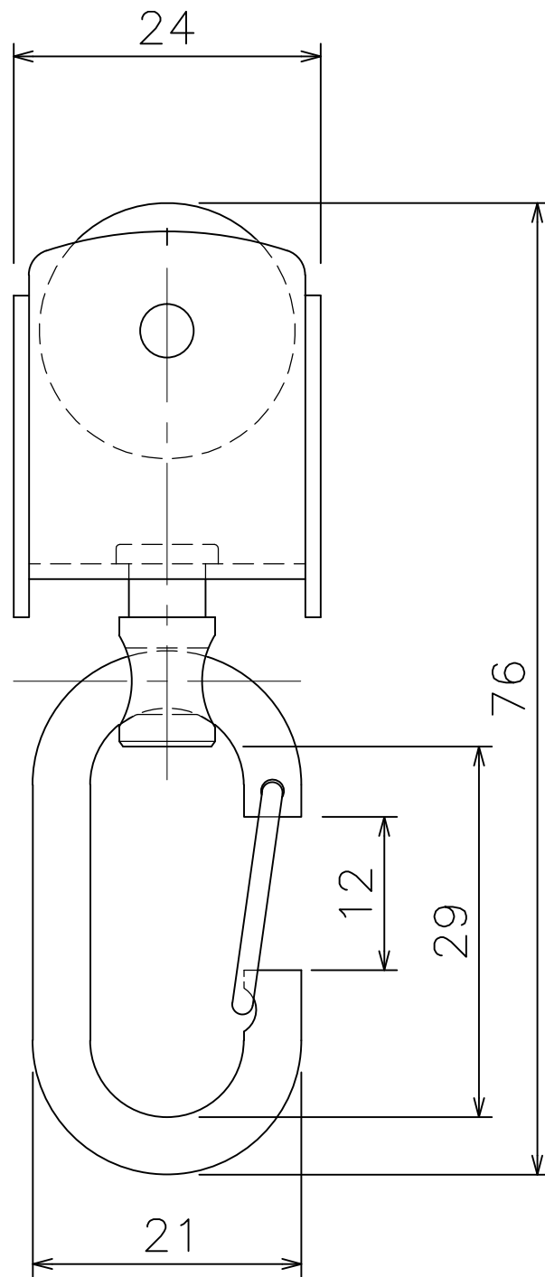
ベンダー ワンタッチランナー (19T12)
