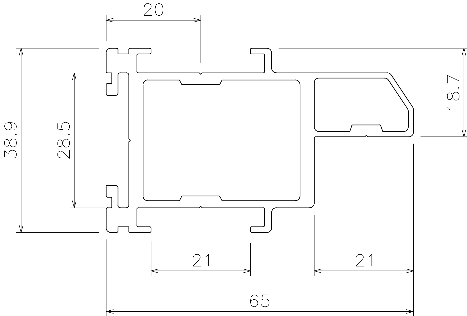
間仕切 サイドポール HG (96S***)
