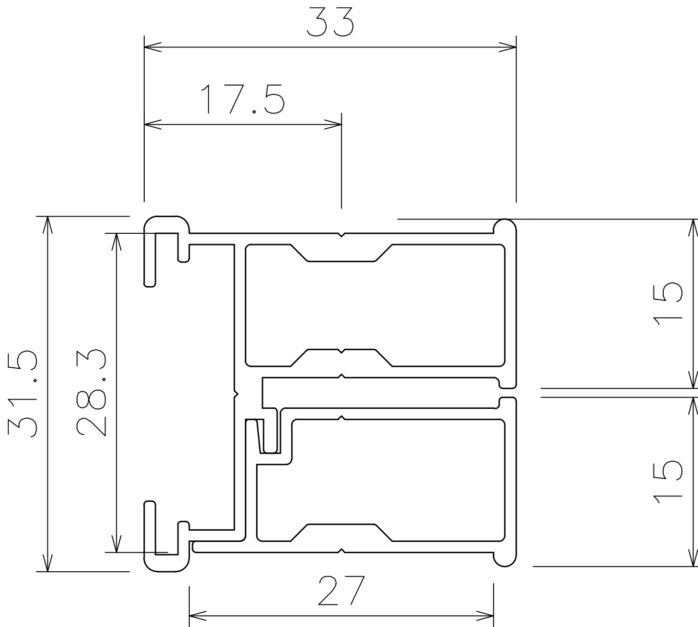
間仕切 サイドポール 挟込 (91S***)
