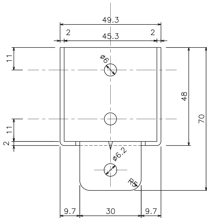
SG ステン壁付けソケット (27T36)
