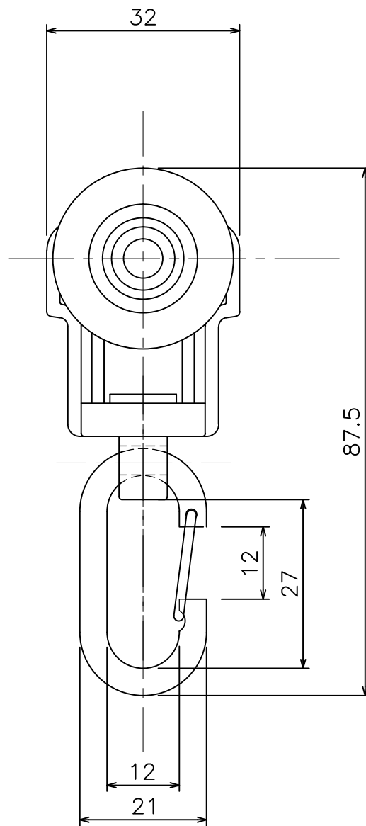
SGワンタッチランナー (27T27)
