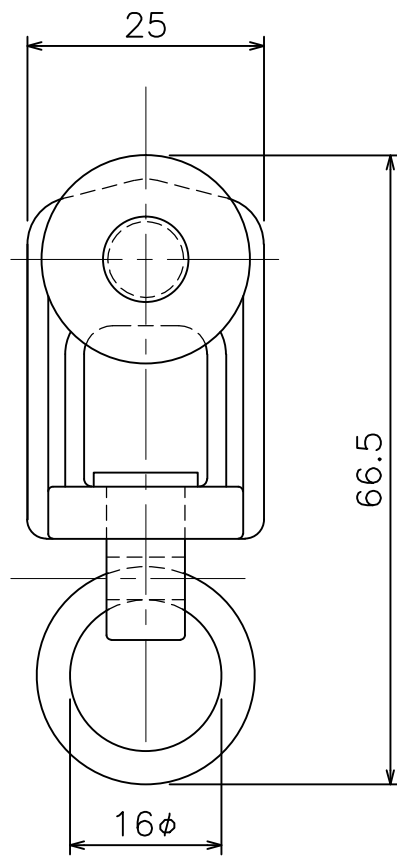
HG ランナー (24T26)
