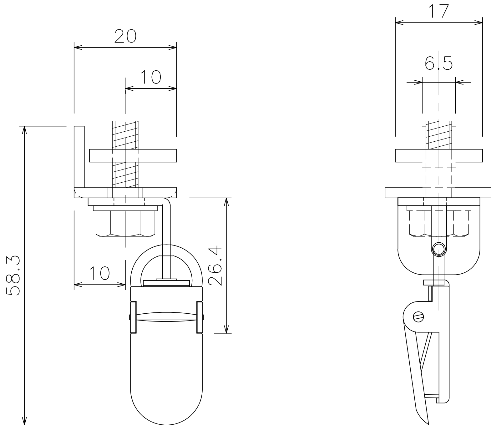
D25 クリッパー付中間ストップ (9T40)
