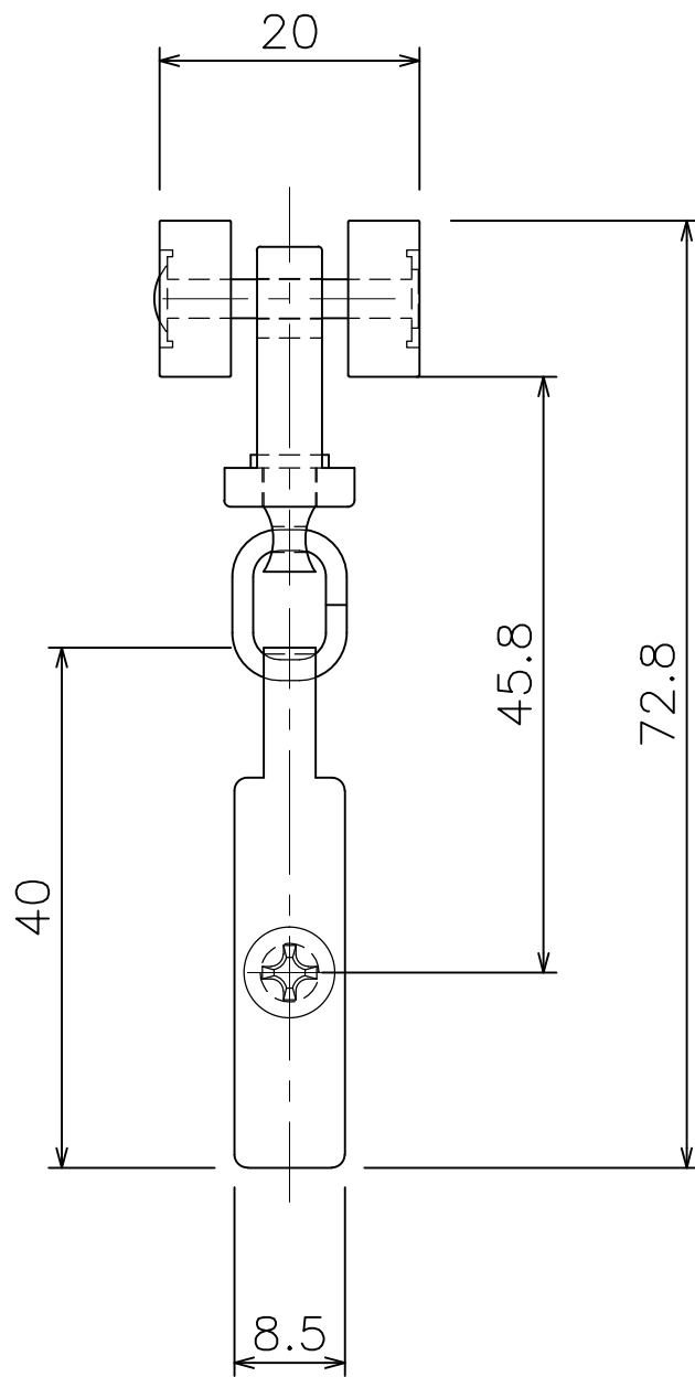
D25 間仕切用ランナー (9T28)
