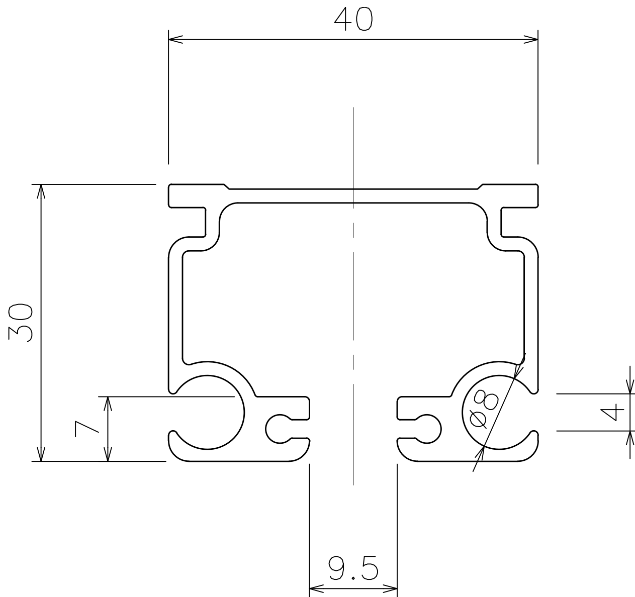
D40隙間シートレール (20L** *-AS)
