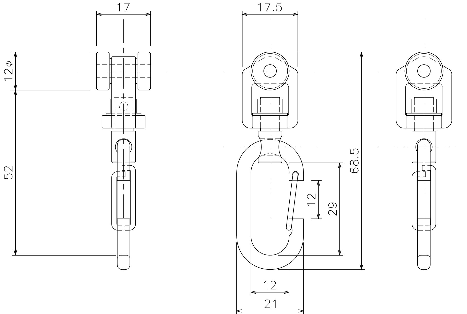
D30 ベアリング入ワンタッチランナー (12T27)
