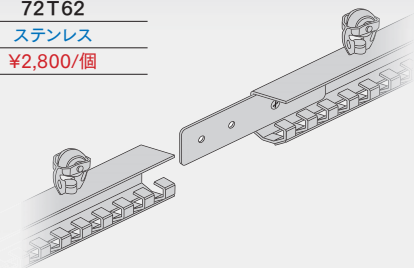
取付ビス付
