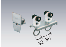
D30片マグネットランナー(片開) 通常ランナータイプ
