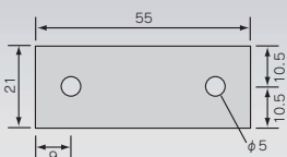
吊棒天井付面寸法図
