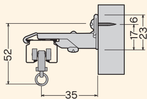
D25・Sブラケット (9T43) スチール/シルバー 100ヶ入 @¥190
