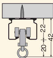
D25天井Sブラケット (9T53) スチール/シルバー 100ヶ入 @¥190
