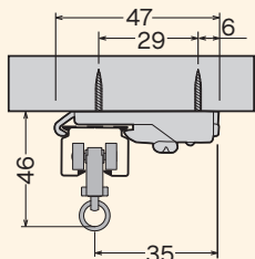
D25天井Sブラケット (9T53) スチール/シルバー 100ヶ入 @¥190
