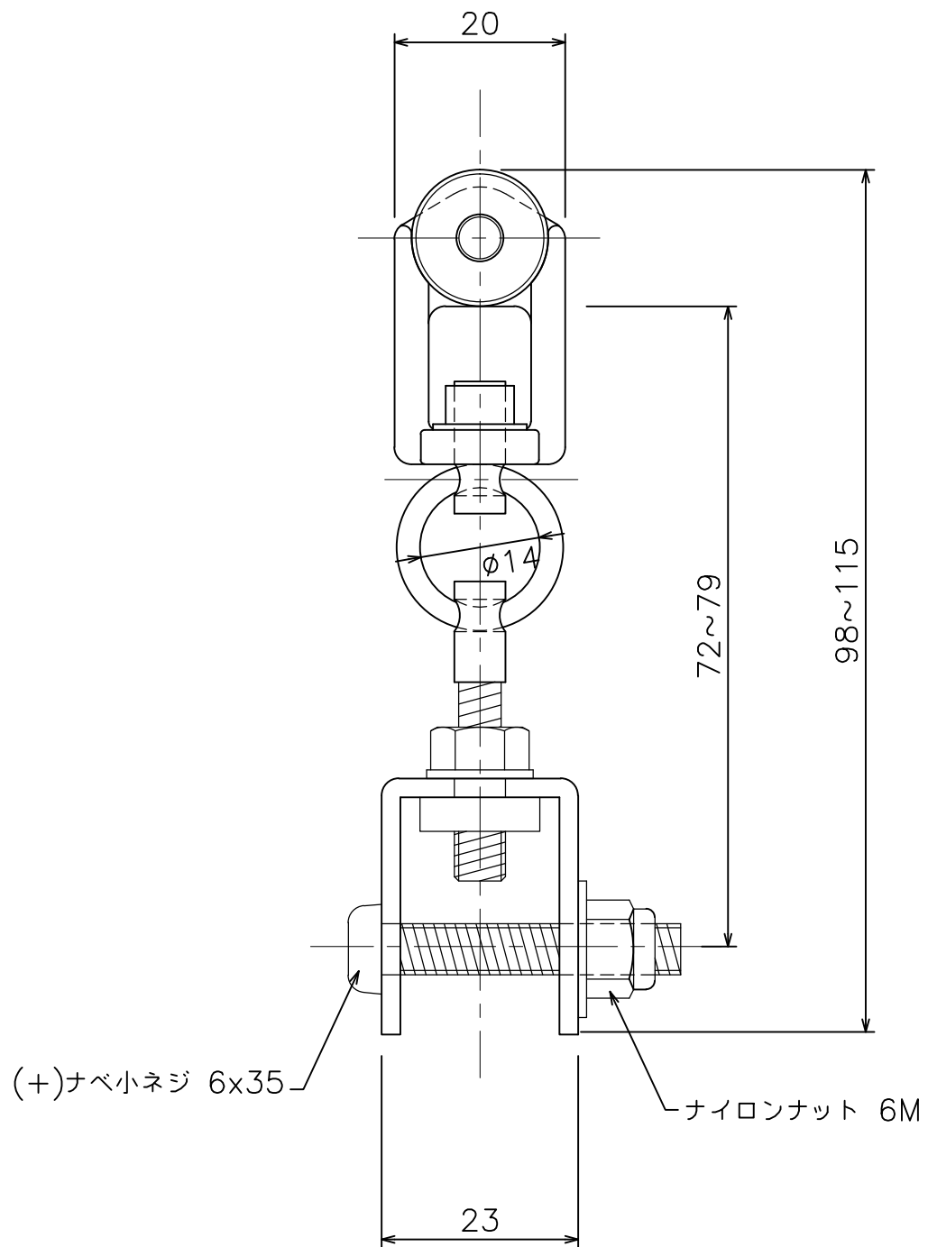
D40 間仕切用ランナー (15T28)
