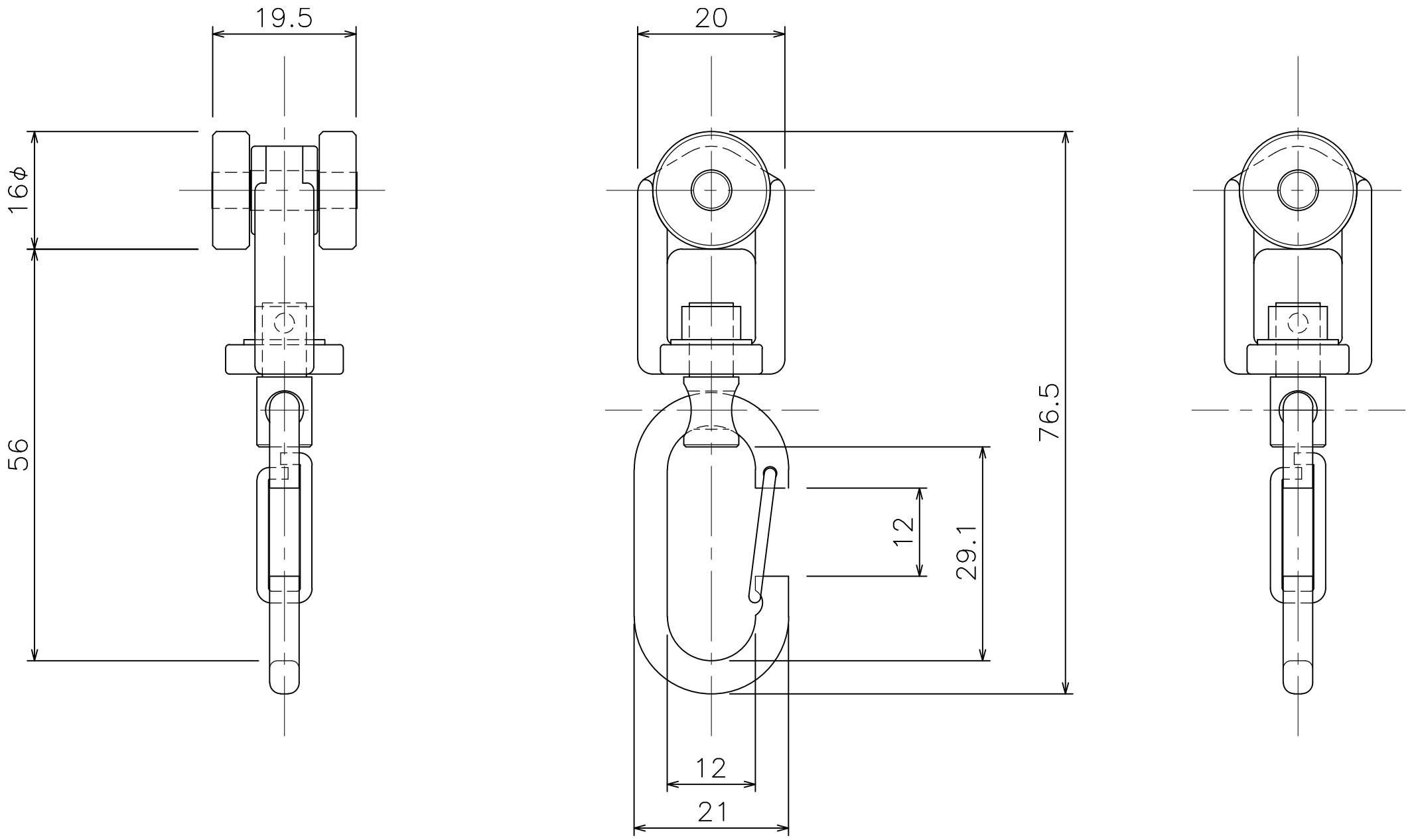
D40 ベアリング入ワンタッチランナー (15T 27)
