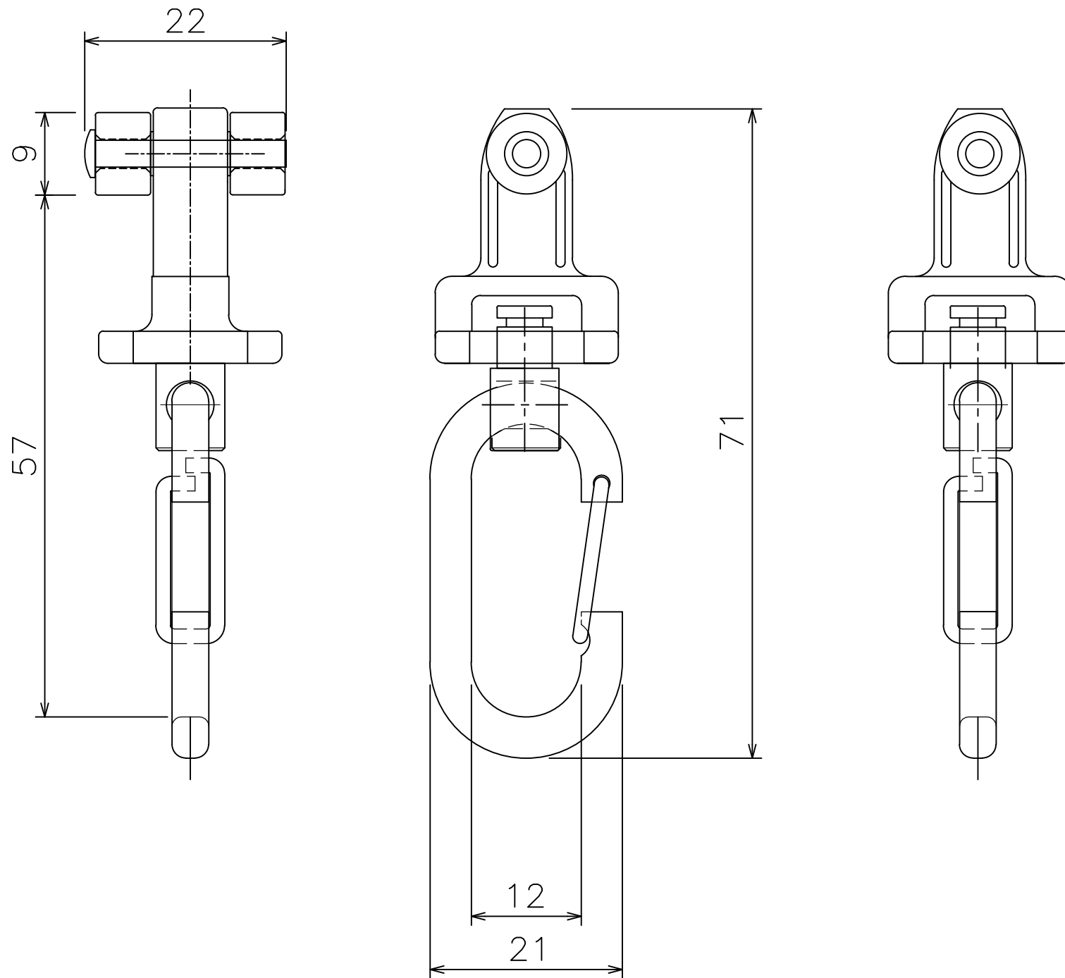
D40 後付ワンタッチランナー(15T20)
