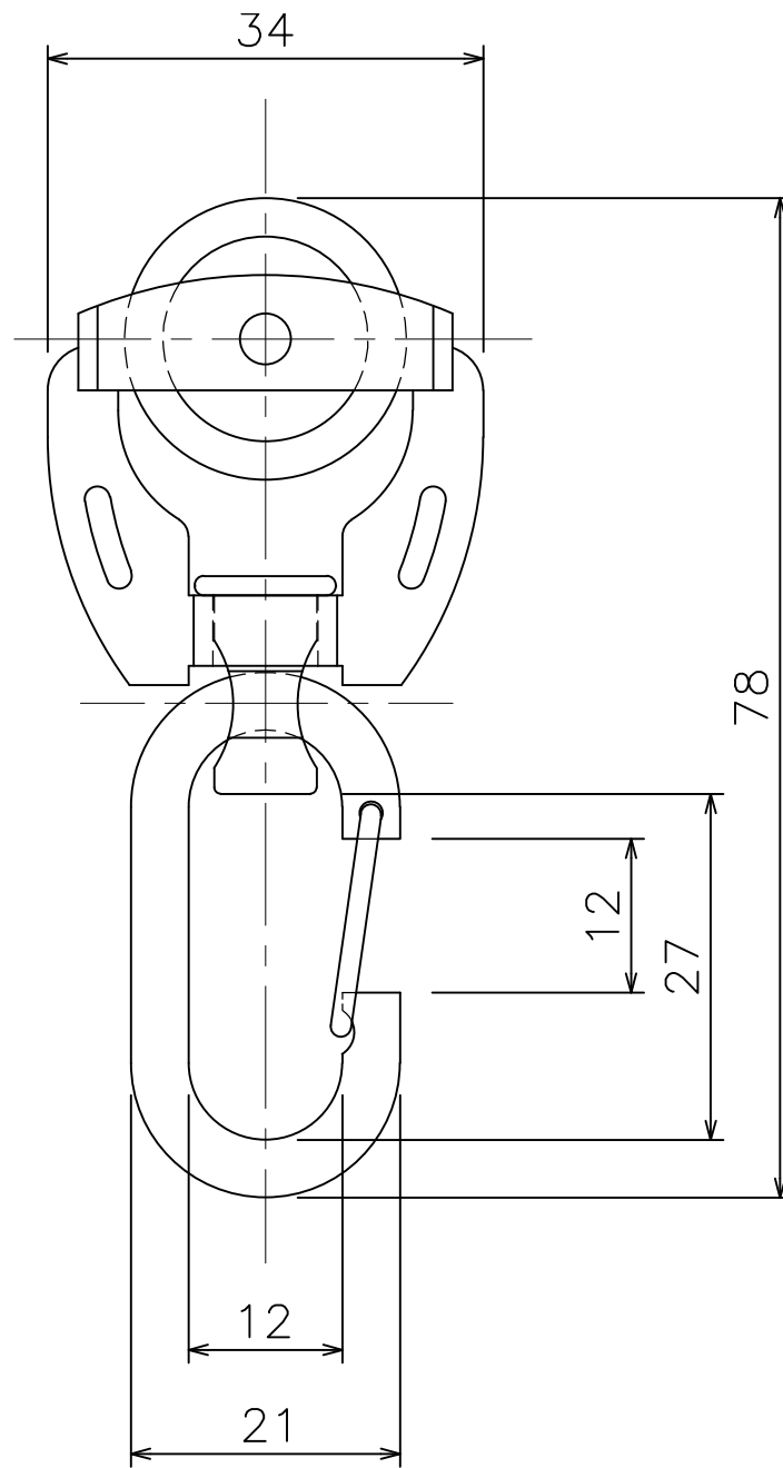
D40 ステン特殊ワンタッチランナー(25T27)
