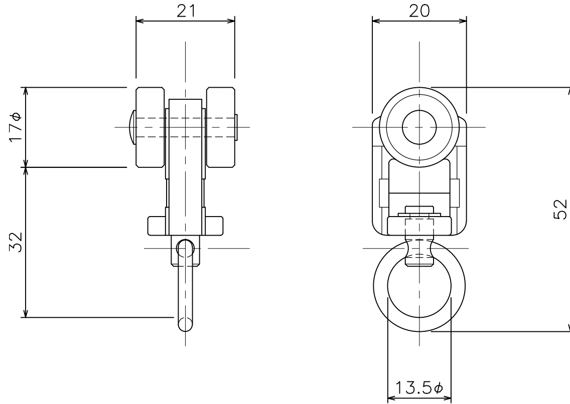
D40 ステンランナー-A (25T 12)
