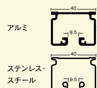
D40レール断面図 (mm)
