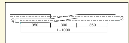
●交叉レール寸法図 (mm)
